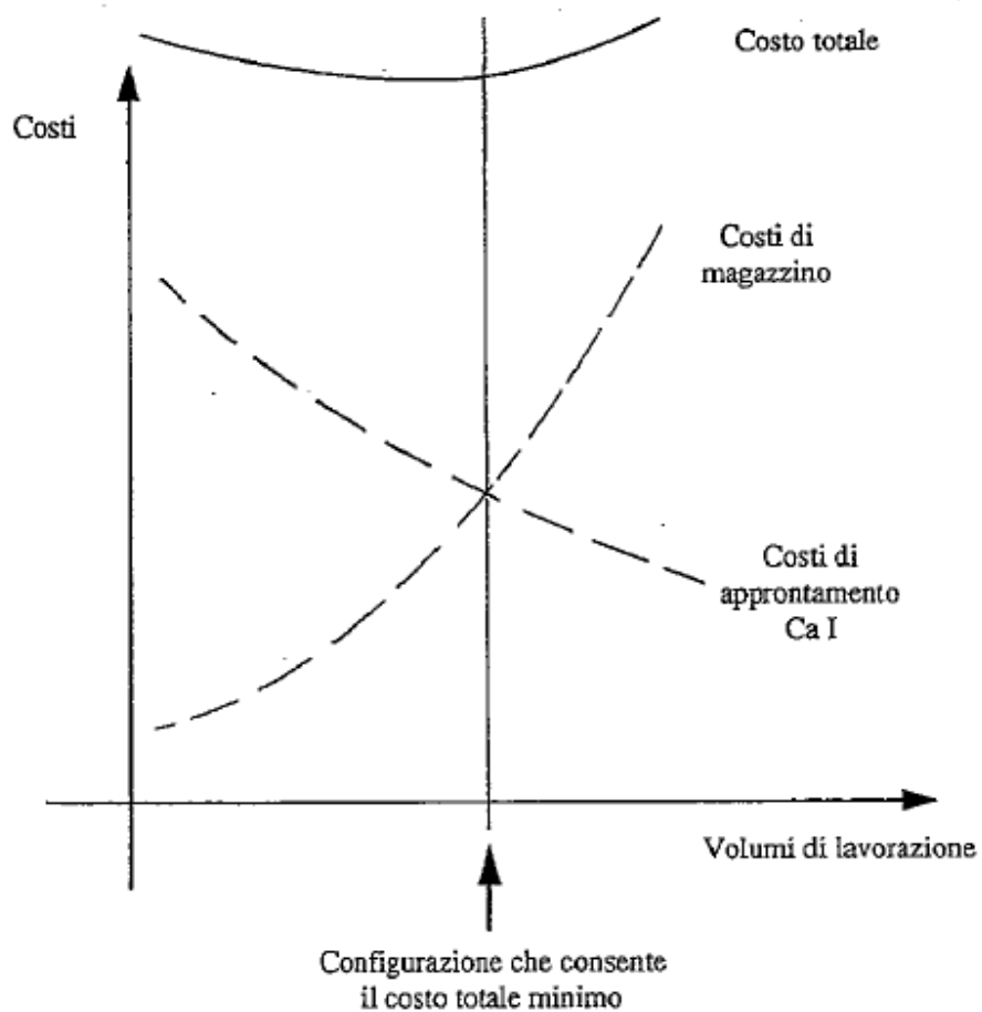
Figura 4.12 - I costi complessivi di fabbricazione di un lotto di prodotti, come sommatoria dei costi di approntamento del lotto e dei costi di magazzino
